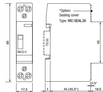
fig. 3. Dimensions (mm)
