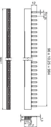
fig. 1. Abmessungen (mm)
