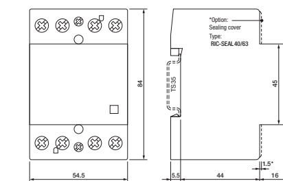
fig. 3. Dimensions (mm)
