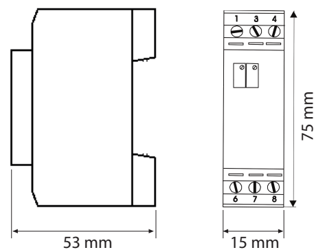
fig. 1. Abmessungen (mm)
