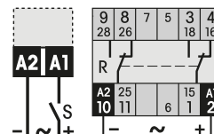
fig. 2. Wechselstrom-Schaltzyklen
