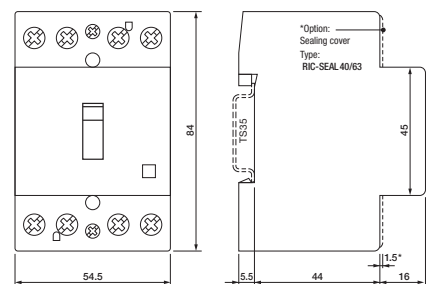
fig. 3. Abmessungen (mm)
