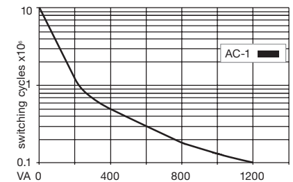
fig. 3. Gleichstrom-Grenzlastkurve
