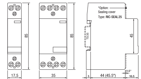
fig. 2. Abmessungen (mm)
