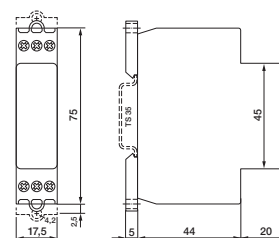
fig. 2. Abmessungen (mm)
