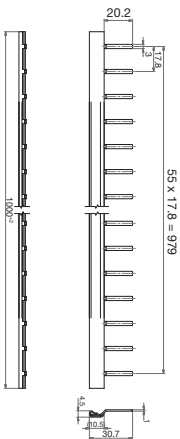
fig. 1. Dimensions (mm)
