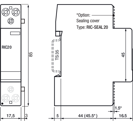
fig. 3. Dimensions (mm)
