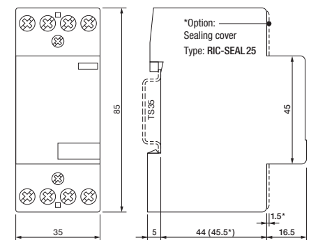
fig. 3. Dimensions (mm)
