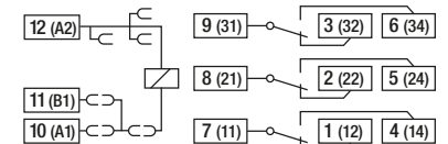
fig. 1. Wiring diagram
