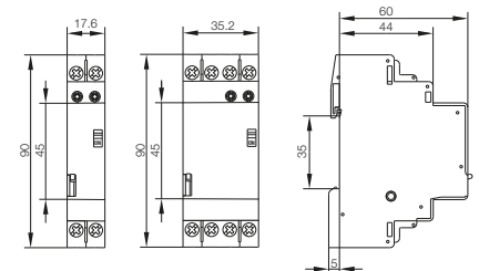
fig. 3. Abmessungen (mm)
