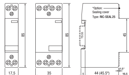
fig. 2. Abmessungen (mm)
