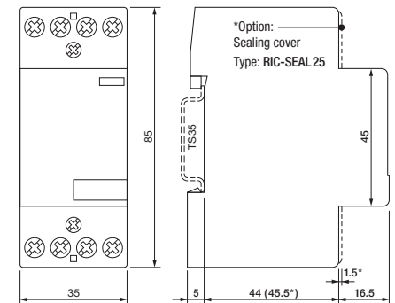
fig. 3. Abmessungen (mm)
