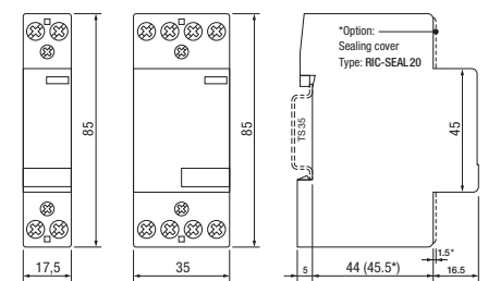
fig. 3. Dimensions (mm)
