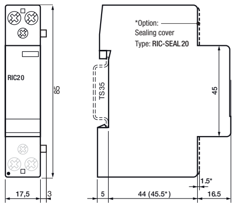
fig. 3. Dimensions (mm)
