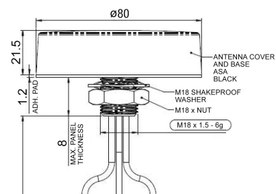
fig. 1. Dimensions (mm)
