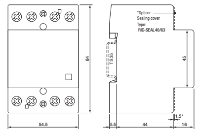
fig. 3. Dimensions (mm)
