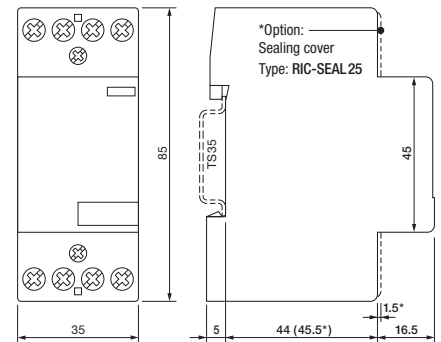
fig. 2. Abmessungen (mm)
