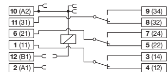
fig. 1. Wiring diagram
