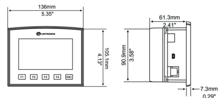
fig. 1. Abmessungen (mm)
