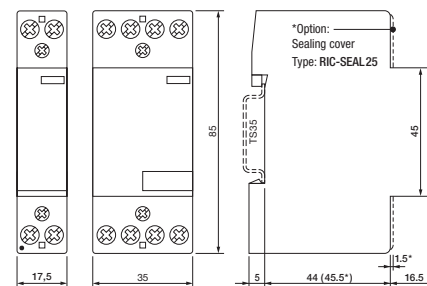
fig. 2. Abmessungen (mm)
