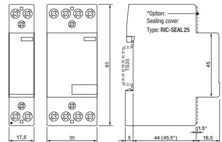
fig. 2. Abmessungen (mm)
