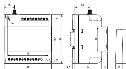
fig. 3. Dimensions (mm)
