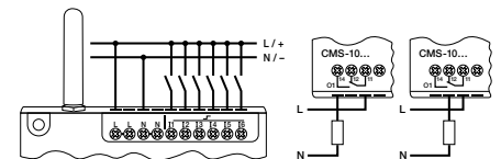
fig. 2. Pouvoir de coupure maximum RZ
