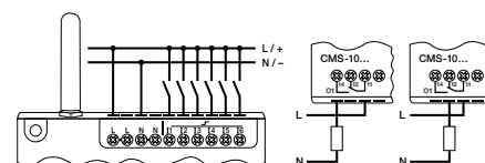
fig. 2. Pouvoir de coupure maximum RZ
