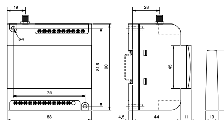
fig. 3. Mått (mm)
